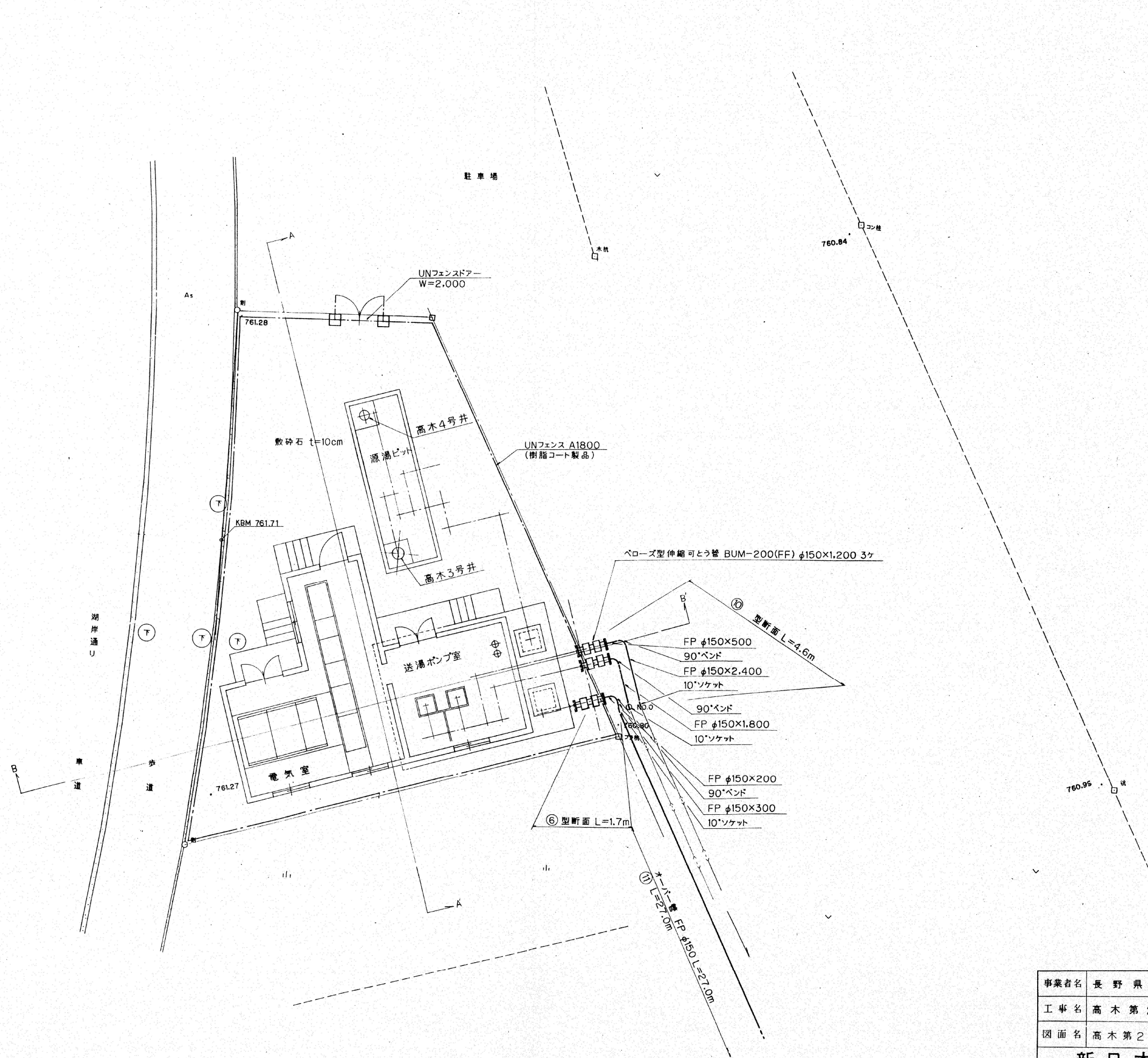
高木第2源湯場施設平面図 S = 1:100
