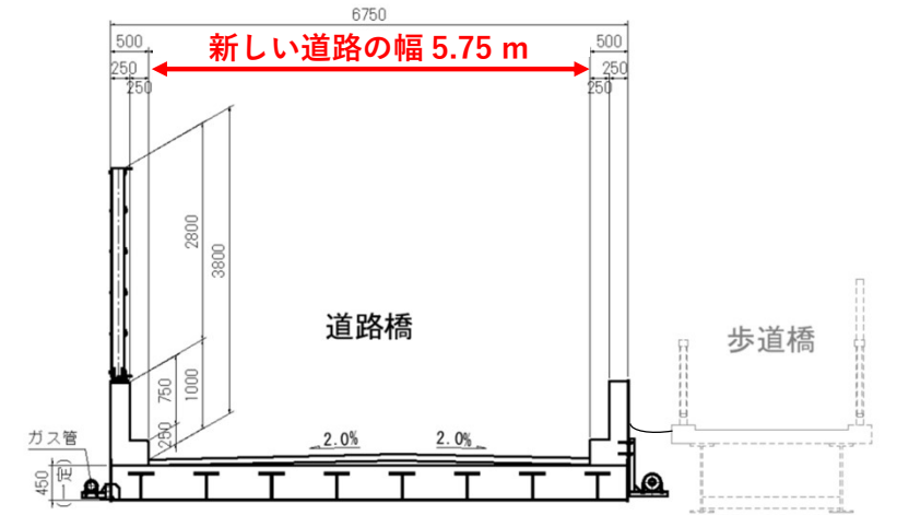
断面図
