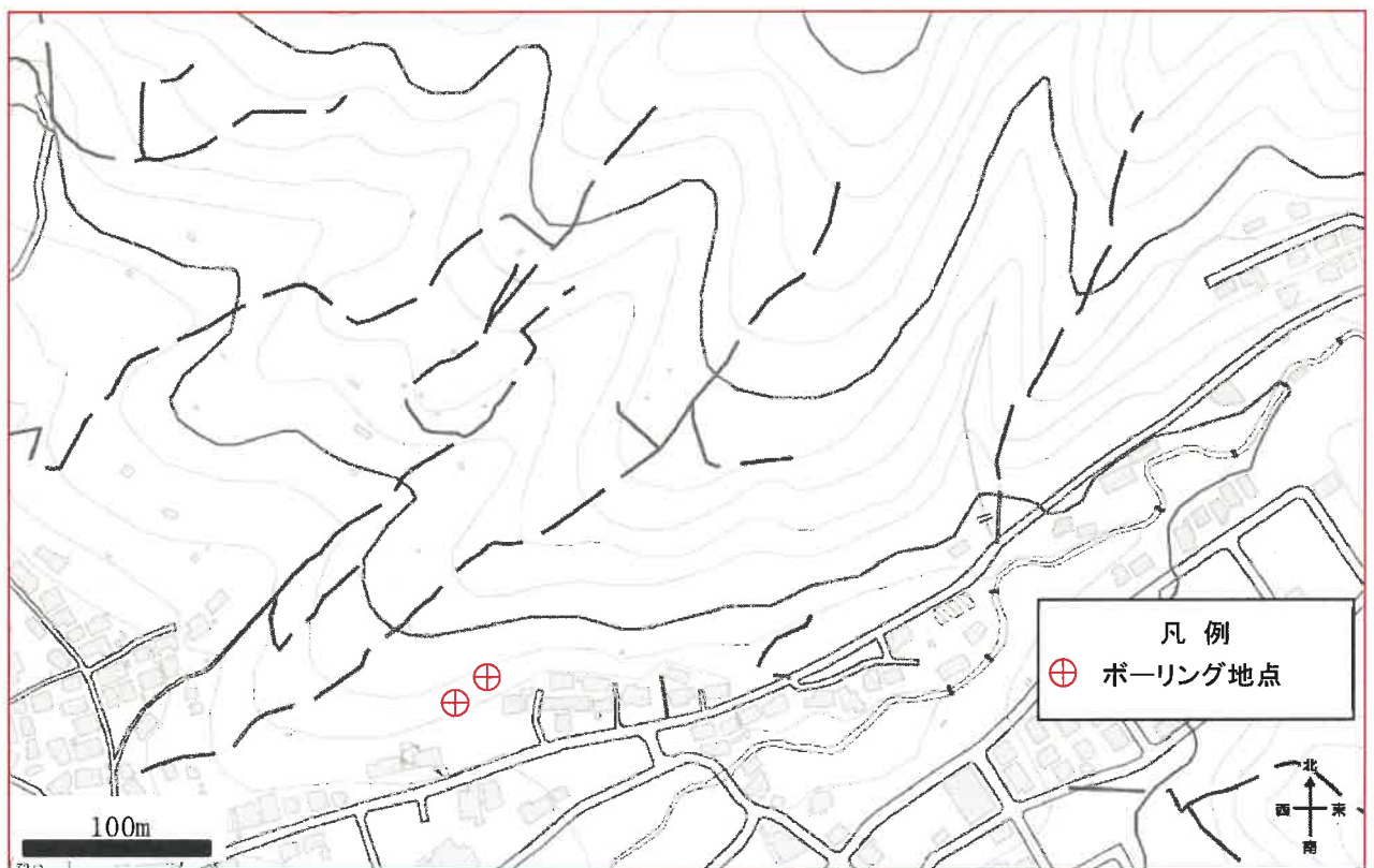
図2 詳細位置図（ボーリング調査）
